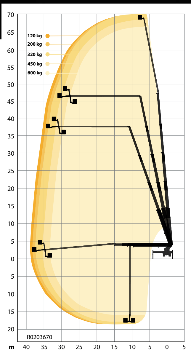
Diagramas presentados con cesta estándar y rotación de la cesta estándar. Pueden existir variaciones. * dependiendo del chasis
